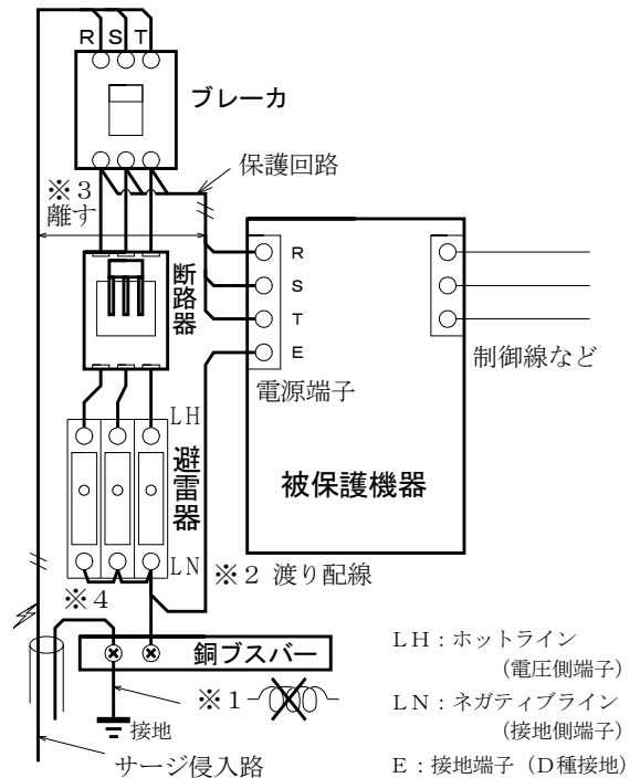
配線例 SG-201-1を3台連結した場合
